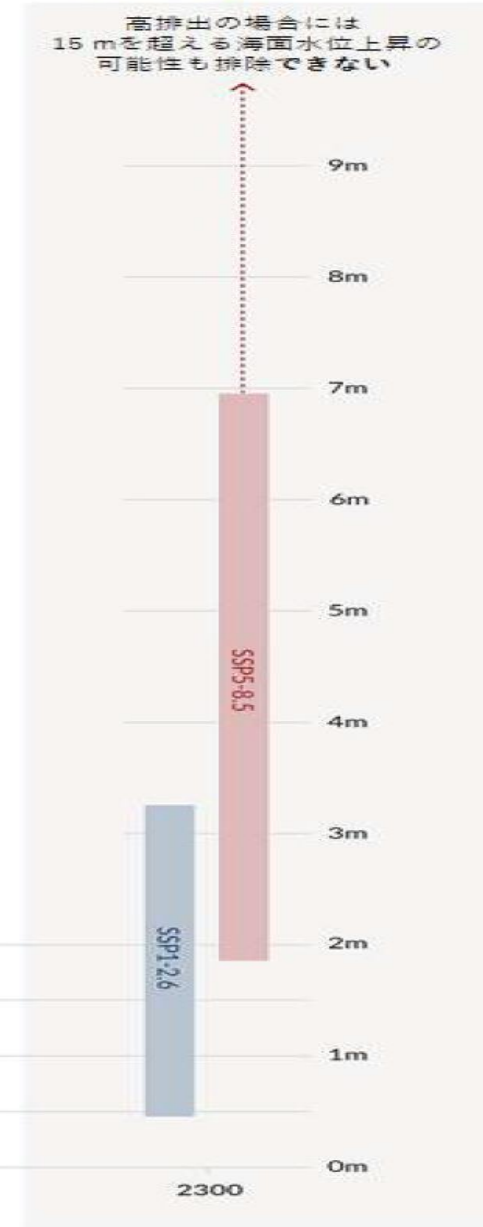
e) 1900年を基準とした 2300年の世界平均 海面水位の変化
